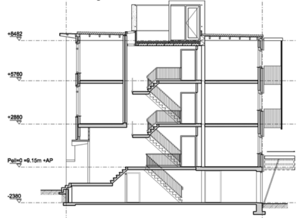
doorsnede trappenhuis
