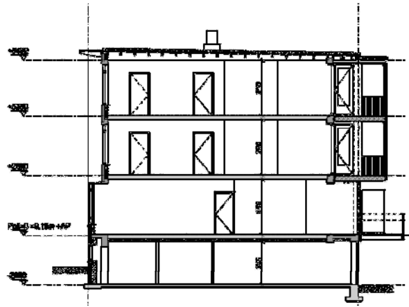
doorsnede woning
