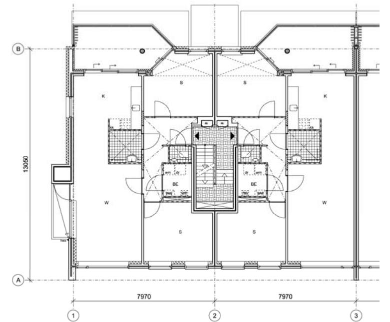
eerste verdieping
