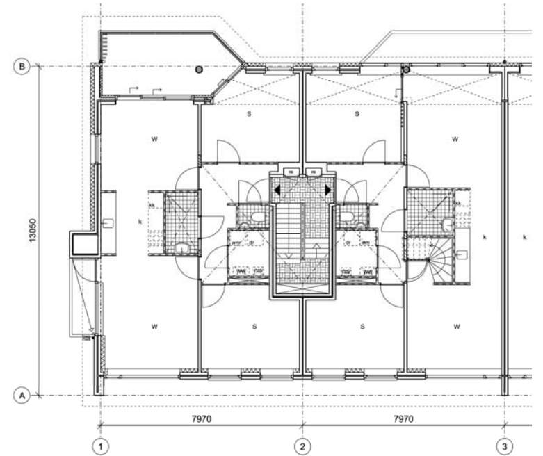
tweede verdieping
